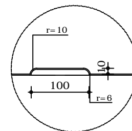
Doorsnede
