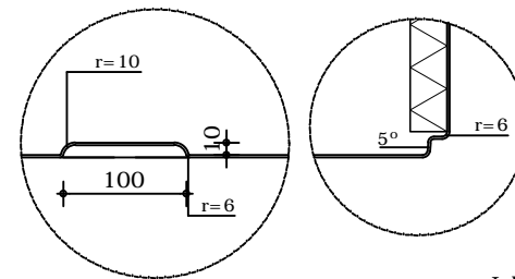
Doorsnede
