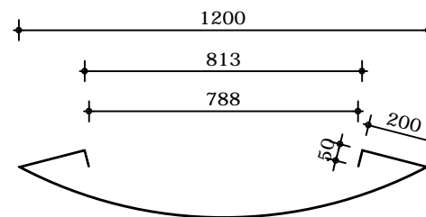
Doorsnede
