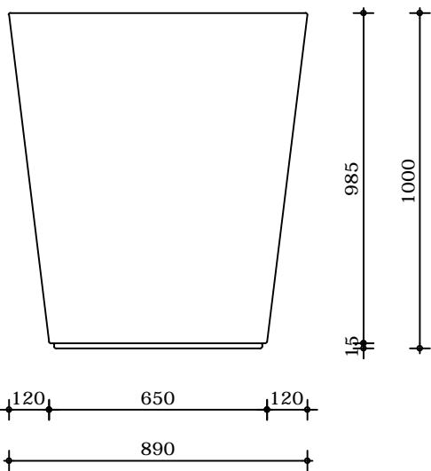
Vooraanzicht
