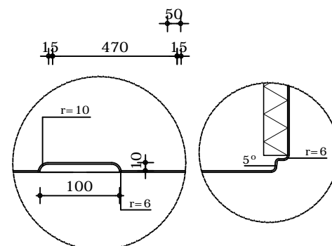
Doorsnede
