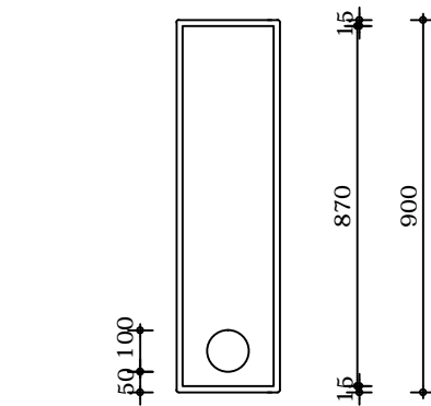
Onderaanzicht 15 220 15 250
