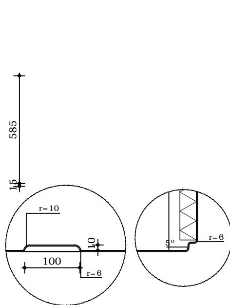
Onderaanzicht
