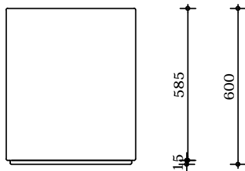
Bovenaanzicht
