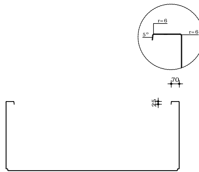
Doorsnede
