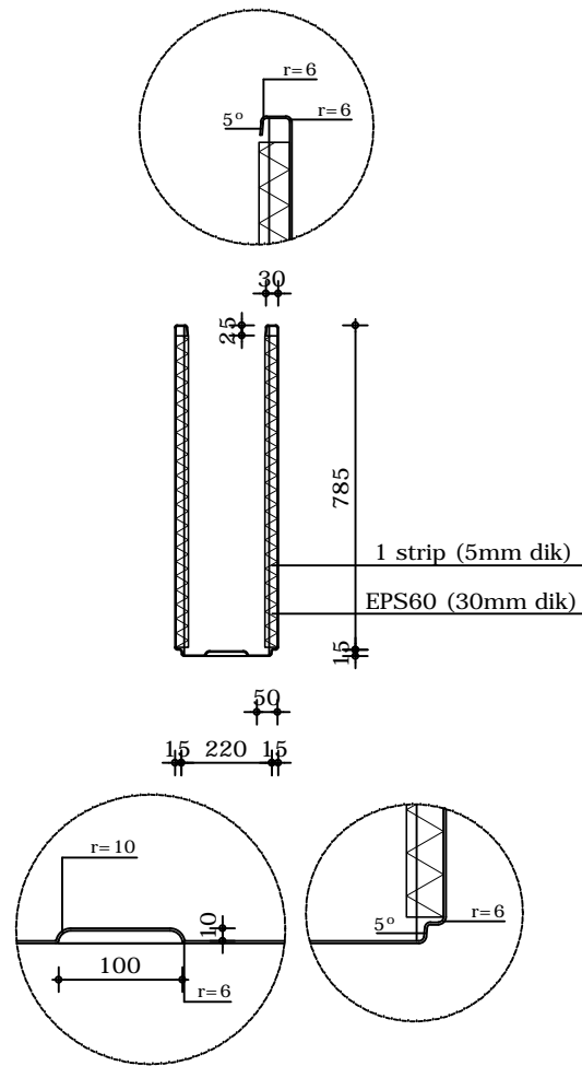
Doorsnede
