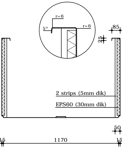
Doorsnede
