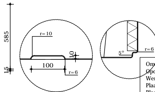
Onderaanzicht
