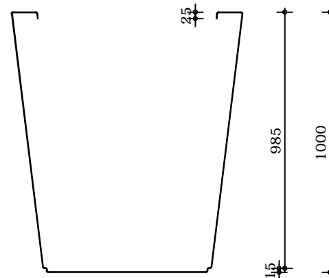
Doorsnede
