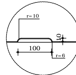
Doorsnede
