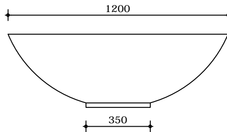
Vooraanzicht
