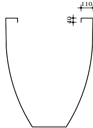
Doorsnede
