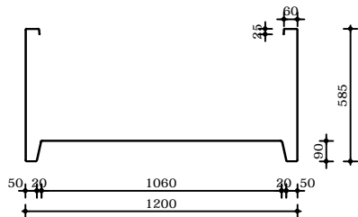
Langsdoorsnede
