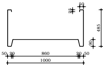
Langsdoorsnede
