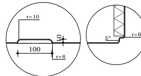
Doorsnede
