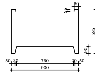
Langsdoorsnede
