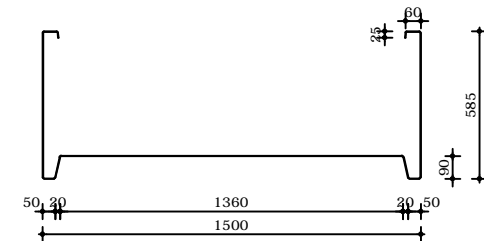
Langsdoorsnede
