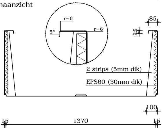
Doorsnede
