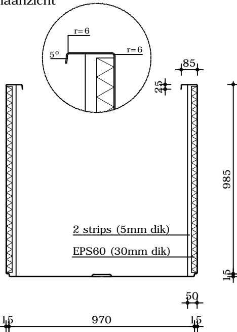
Bovenaanzicht
