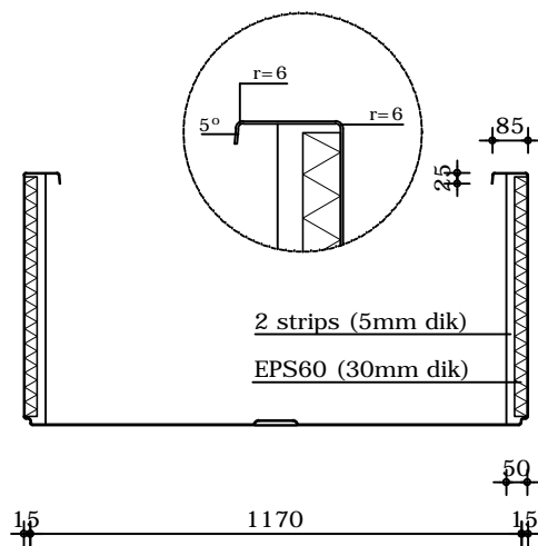
Doorsnede
