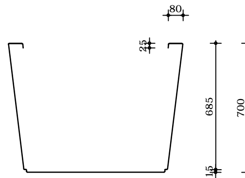
Doorsnede
