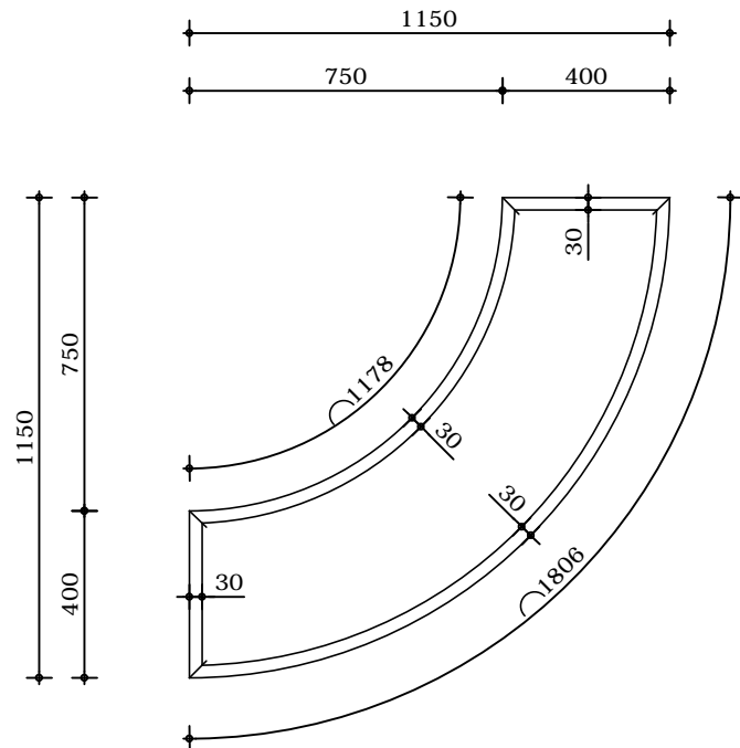
Bovenaanzicht
