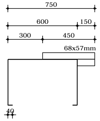
Verticale doorsnede
