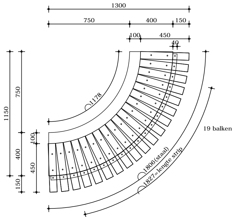
Bovenaanzicht
