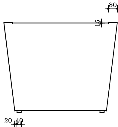
Verticale doorsnede
