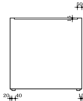
Verticale doorsnede
