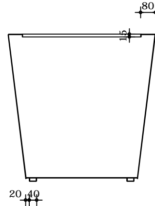
Verticale doorsnede
