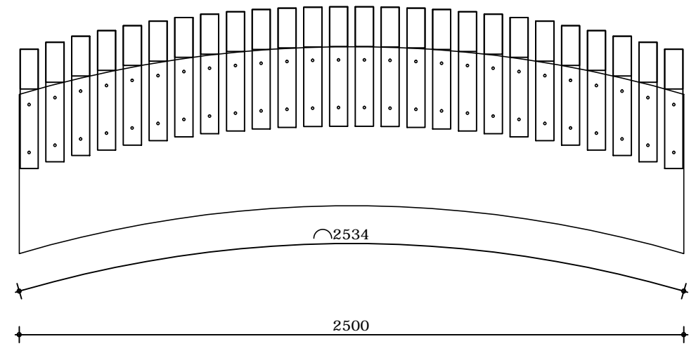
Bovenaanzicht
