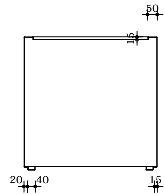
Verticale doorsnede
