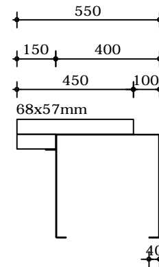
Verticale doorsnede
