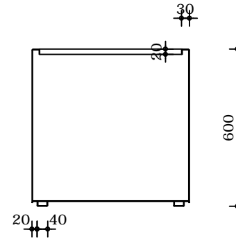
Verticale doorsnede
