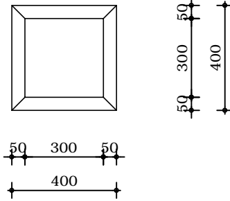
Bovenaanzicht
