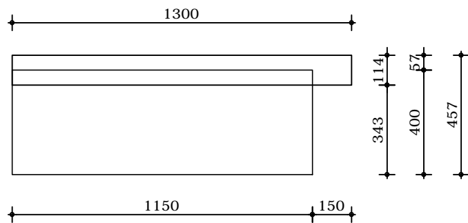
Vooraanzicht
