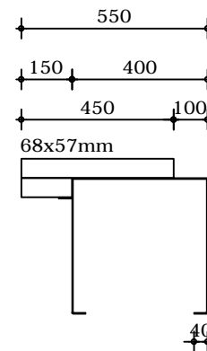
Verticale doorsnede
