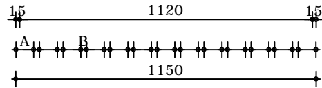
Bovenaanzicht
