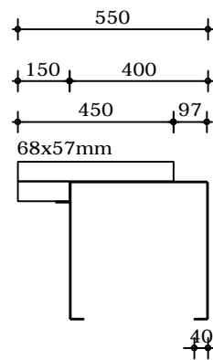
Verticale doorsnede
