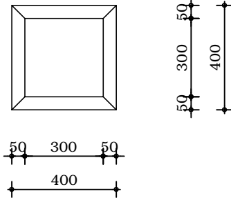
Bovenaanzicht
