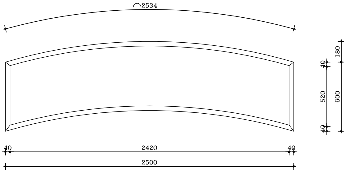
Bovenaanzicht
