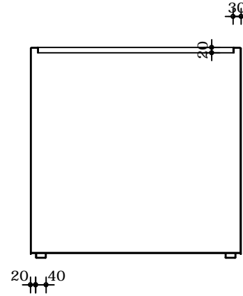
Verticale doorsnede
