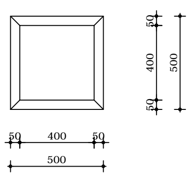
Bovenaanzicht
