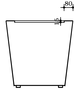
Verticale doorsnede
