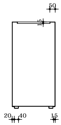
Verticale doorsnede
