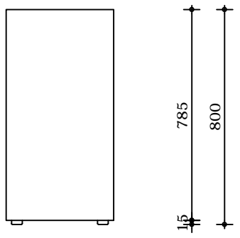
Voorraanzicht
