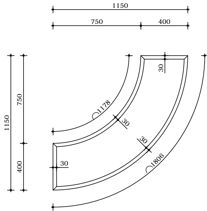
Bovenaanzicht
