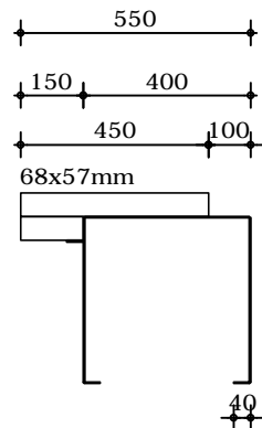
Verticale doorsnede
