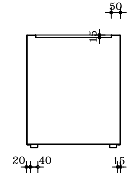
Verticale doorsnede
