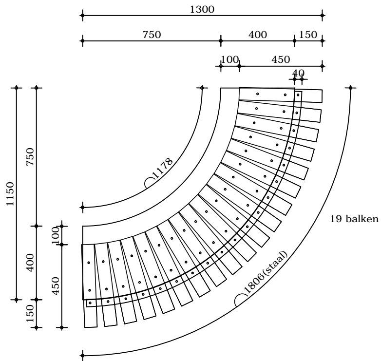
Bovenaanzicht
