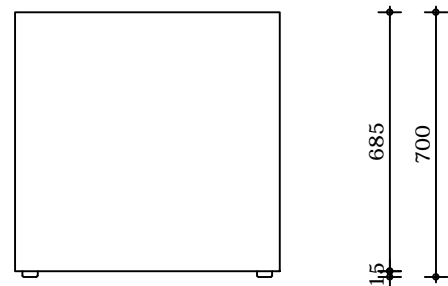
Vooraanzicht
